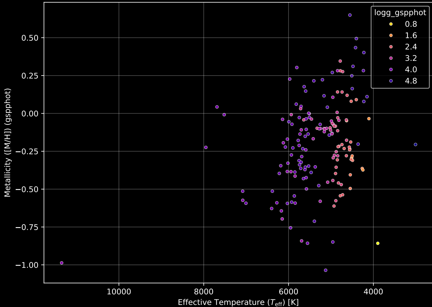
APOGEE DR17 Field: [278-27-O_TESS] Stellar Population Parameters (n= 165)
